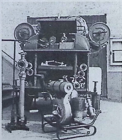
Tragkraftspritzenanhänger
